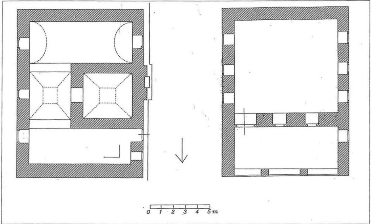
Mektebin zemin ve üst kat planları
