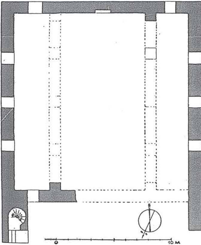
Kumluk (Ağalar) Camii planı...
