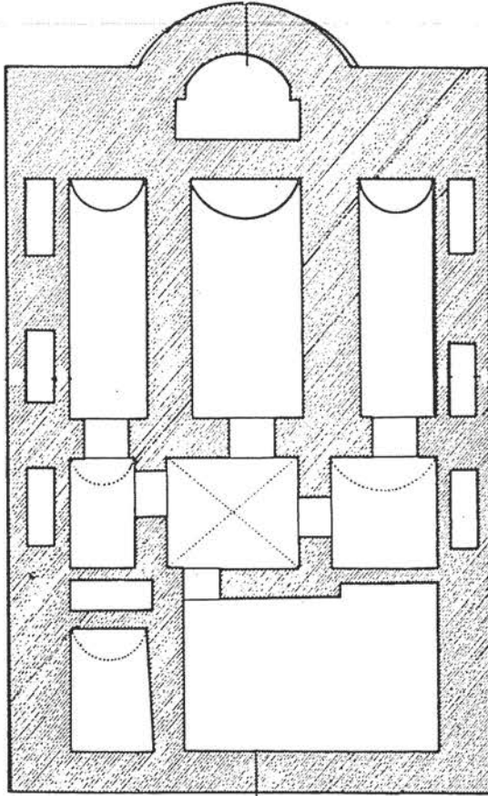
Tiyatro yanındaki kilise alt yapısının planı.
