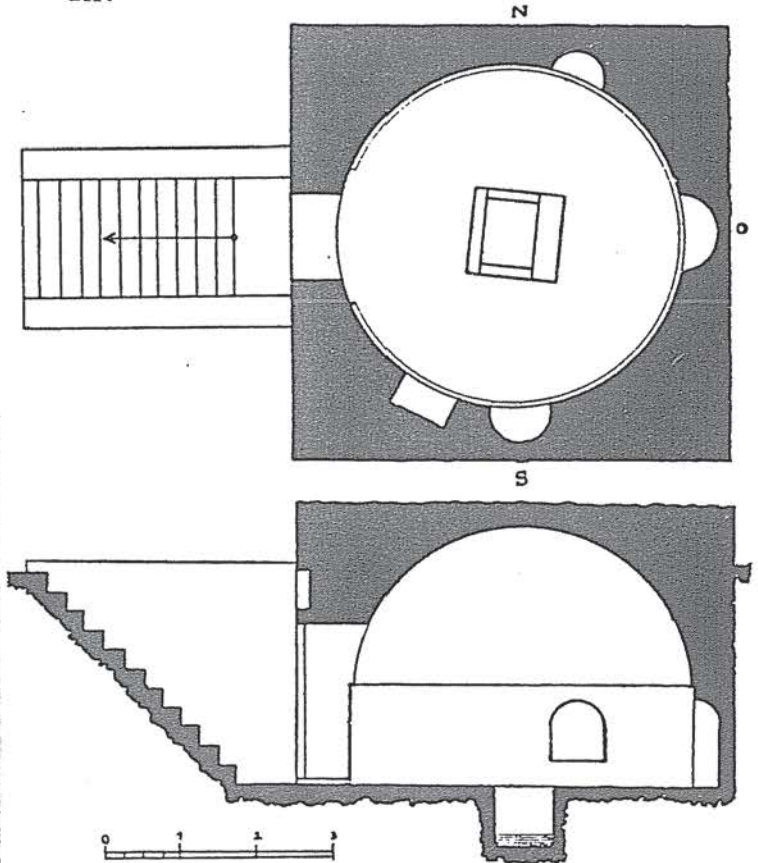
Böcek Ayazması plan ve kesiti.
