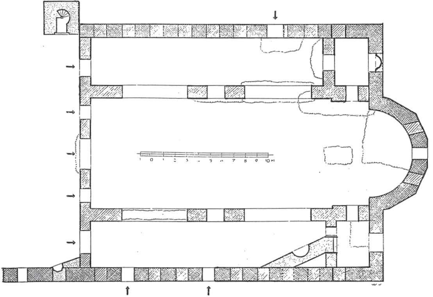
Ayasofya Kufesi plan ve kesiti...
