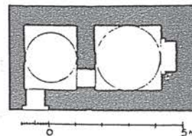
Yenişehir kapı yanındaki küçük hamam'ın planı.
