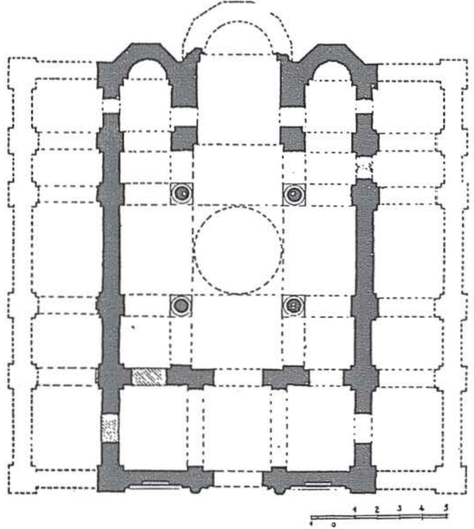
İstanbul kapı yakınındaki kilisenin planı.
