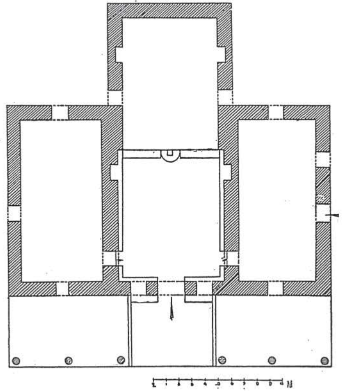
• Orhanbey imaret plâni
