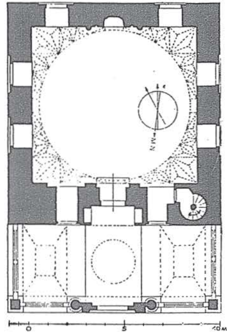
Mahmut Çelebi Camii planı.
