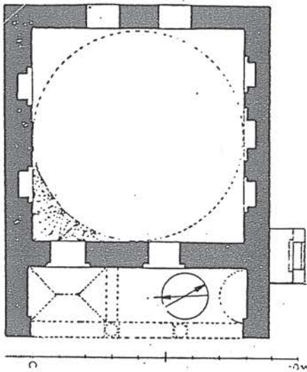
Hacı Özbek Camii planı.
