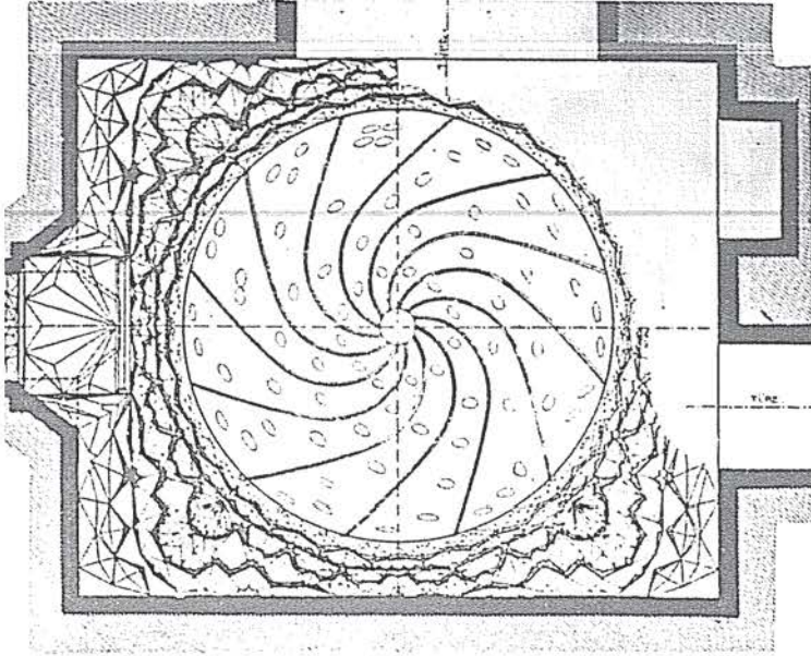
İsmail Bey Hamamı plan ve kesitleri.
