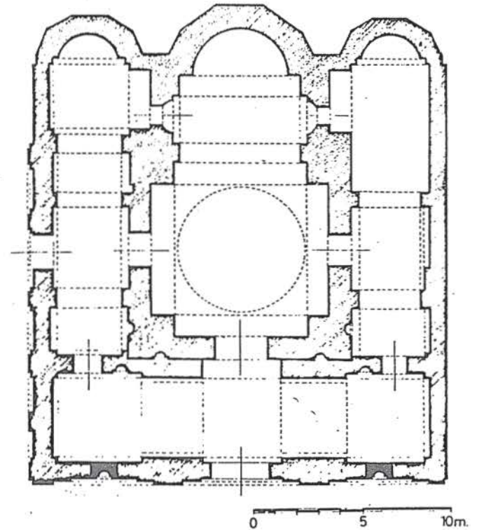
Yenişehir kapı yakınındaki kilisenin planı...
