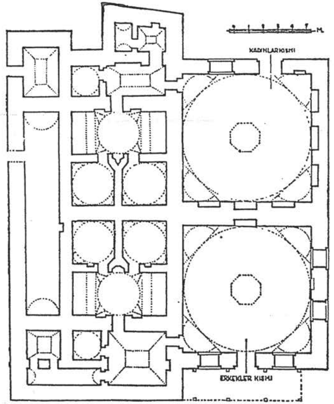
Büyük Hamam Planı.
