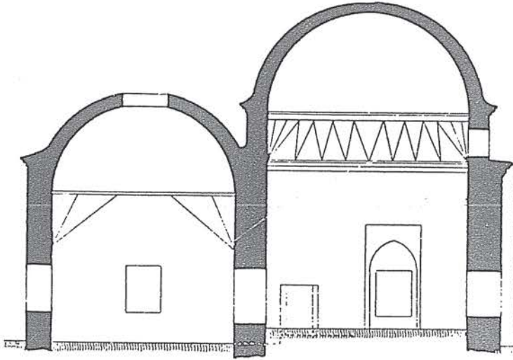
Candarlı Hayrettin Paşa Türbesi plan ve kesiti.
