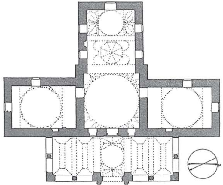
Nilüfer Hatun İmaret plan ve kesiti.
