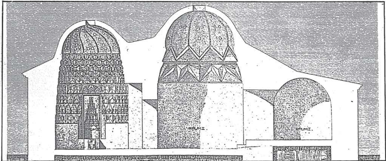
İsmail Bey Hamamı'nın kesiti
