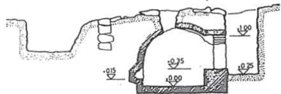
— İznik Çini Fırınları kazısında ortaya çıkan bir fırının plan ve kesiti...
