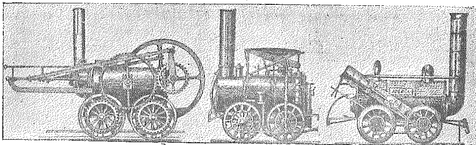
١٨٢٨ ده امريكاده ايشايان ايلك اوقوموتيف ١٨٢٩ سنه سنده امريكاده ايشايان ايلك لوقوموتيف ١٨٥٣ تاريخنده انكلترده ايشايان ايلك لوقوموتيف
