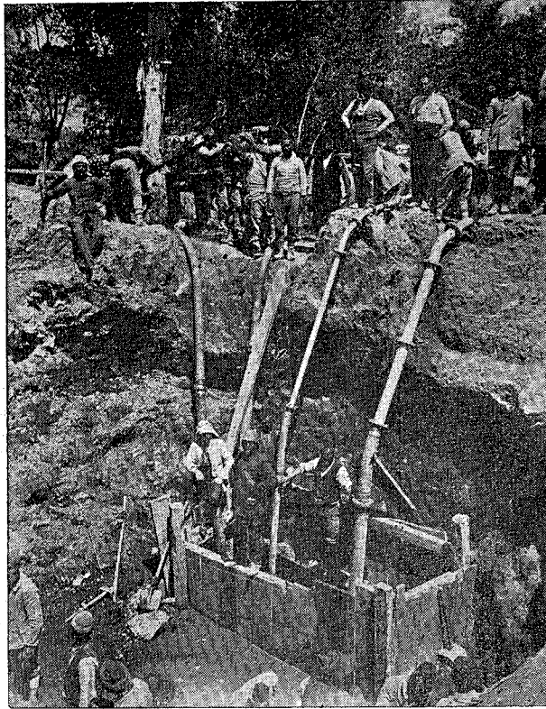
آنقره - سیوس خطلی اوزرنده بویوک رکونپزی تملی حفر ایدیلر ایکن ... ( اشبو فوطوغرافی قارغلمزدن مهندس حسین یعقوب بک طرفدن اهدا بیورلمشدر )
