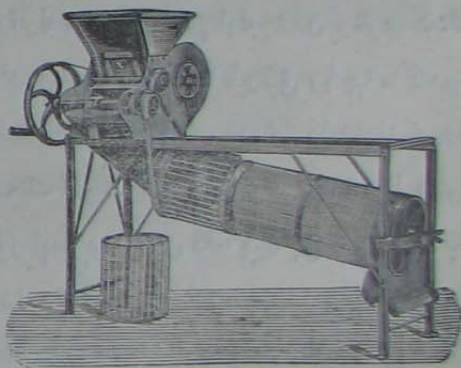
( قابور ماکنه سی )
