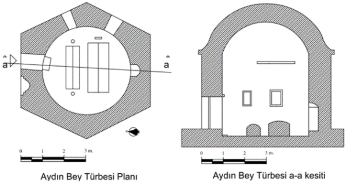
Çizim 1: Aydın Bey Türbesi Plan ve Kesit Çizimi
