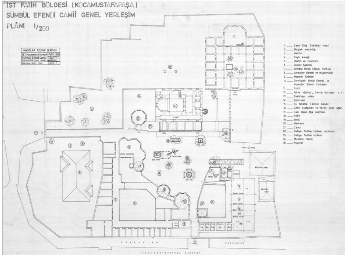
Şekil 1 Vaziyet planı (Vakıflar İstanbul I. Bölge Müdürlüğü Arşivi, Çizen E. Üçer, N. Olgun, S. Nakşibendi).
