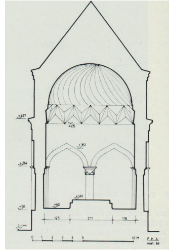
Plan 1-2. Devlet Hatun Türbesi'nin planı ve kesiti (Ayverdi'den)
