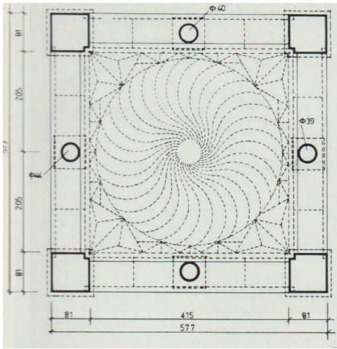
Plan 1-2. Devlet Hatun Türbesi'nin planı ve kesiti (Ayverdi'den)
