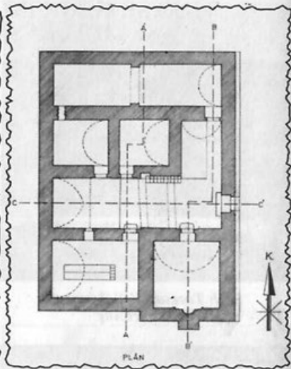
Kayseri, İncesu'da Şeyh Turesan Zaviyesi Planı (Çizen Tevfik Elkovan)
