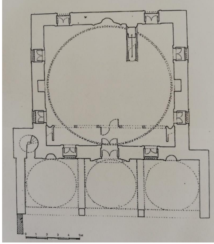
Çizim 1: Nuh Paşa Camii Planı (İ.A. Aslanoğlu'dan)
