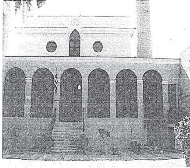
Fotoğraf 1: Sakız Mecidiye Camisi restorasyon sonrası görünüşü (Foto:Neval Konuk, 2015).
