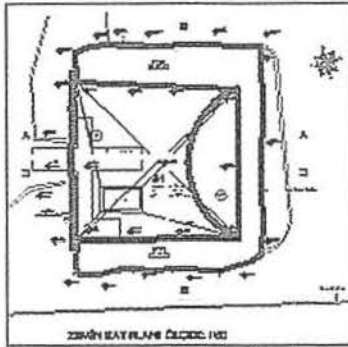
3. Çizim: Doğan Şah Alp Türbesi planı(Mimar Adnan Sevinç)
