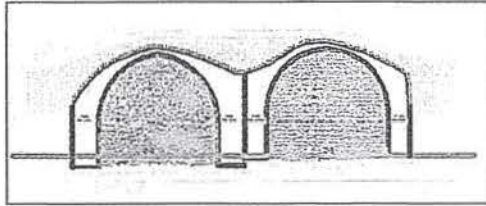
15. Çizim: Eyvan Türbeler kesit (Mimar Adnan Sevinç)
