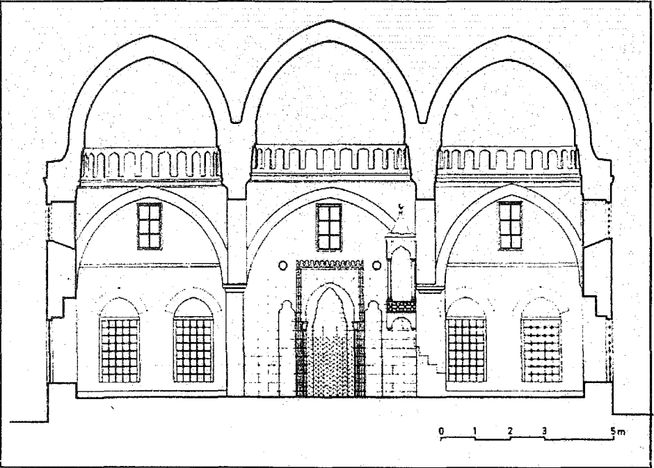
Rizvâniye Câmii kesiti (M. Alper'den)
