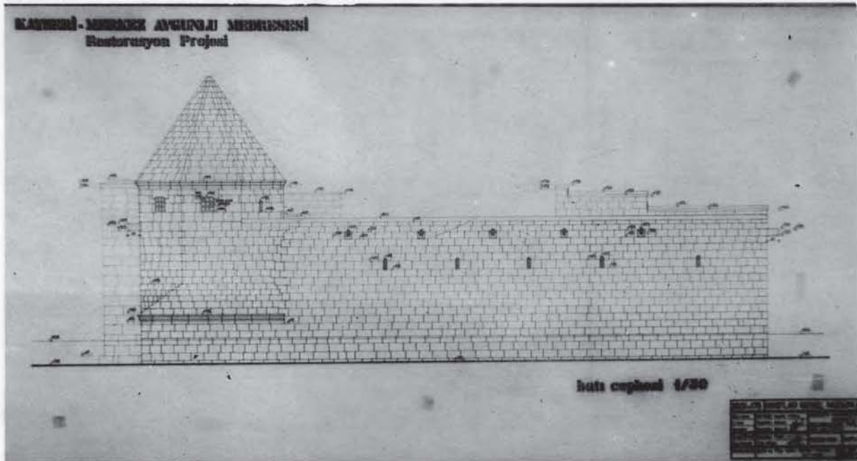
Çizim 9: Restorasyon projesinin batı cephesi.
