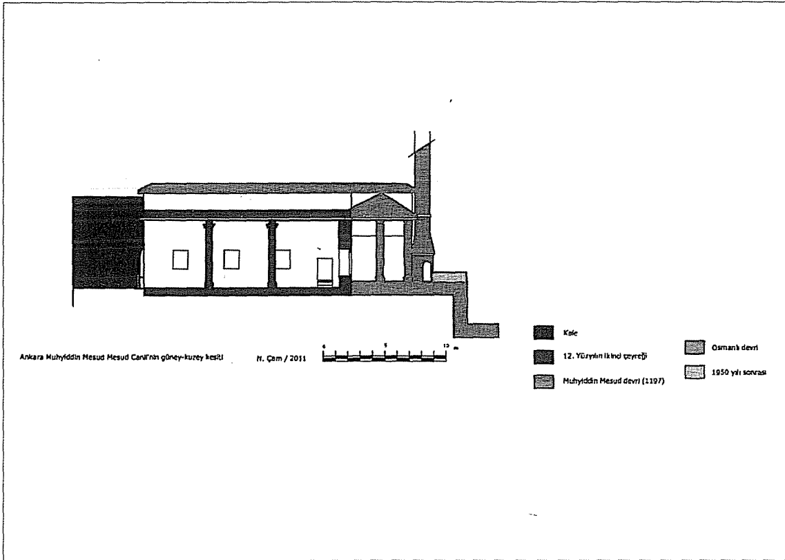
Şekil 4: Muhyiddin Mesud (Alaeddin) Camii'nin güney-kuzey kesiti.
