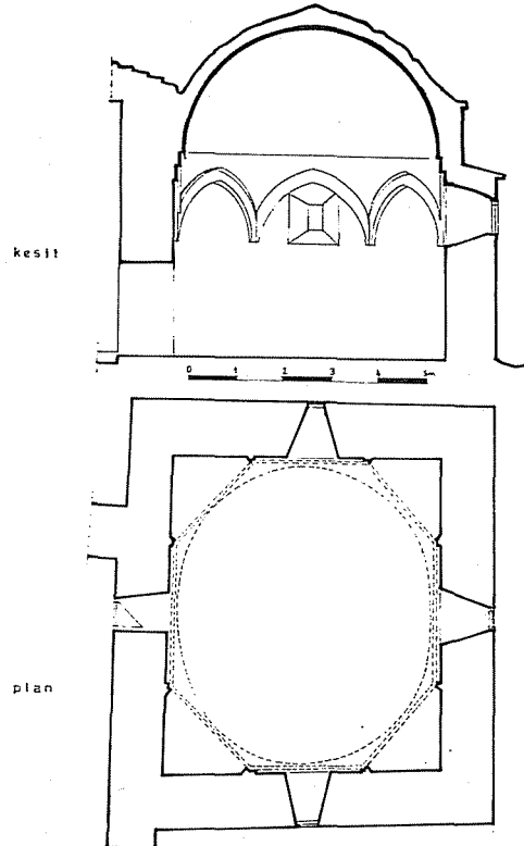
ŞEKİL: 4 Ankara-Sulakyurt Küçük Şamlı Köyü Türbesi plan ve kesiti
