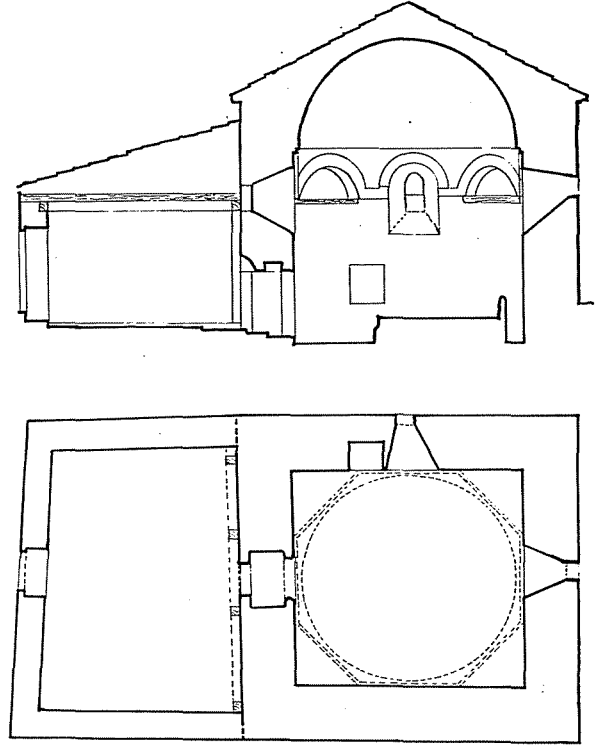
ŞEKİL: 2 Demirşeyh Türbesi plan ve kesiti
