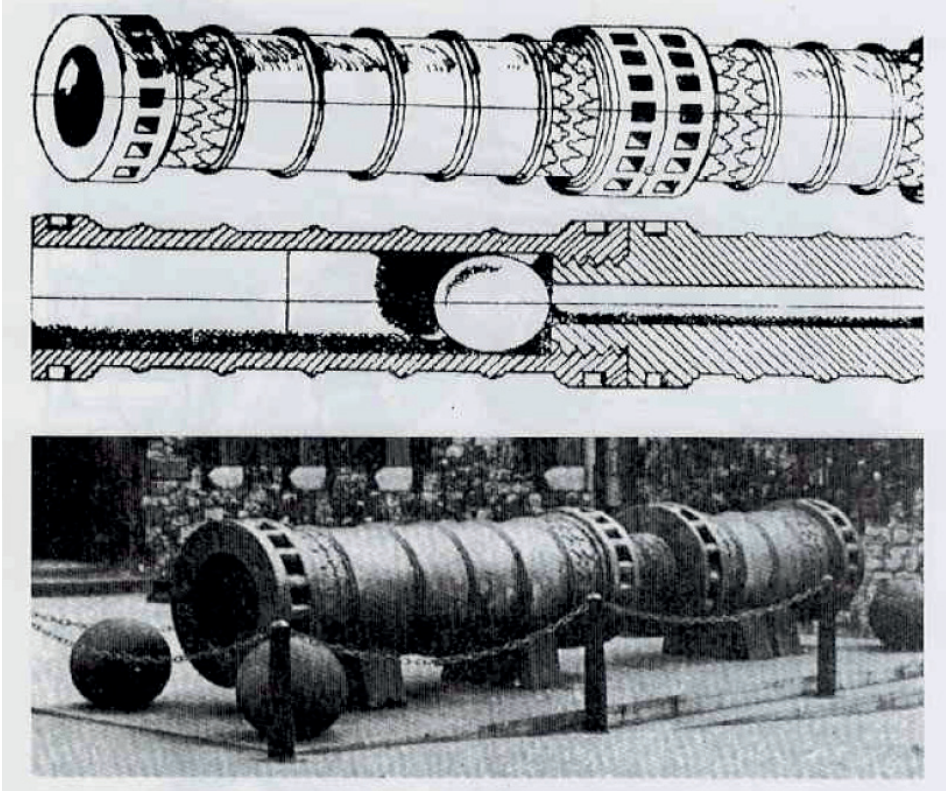
Resim 2. Fort Nelson müzesindeki Şahi topu ve kesiti. 9
