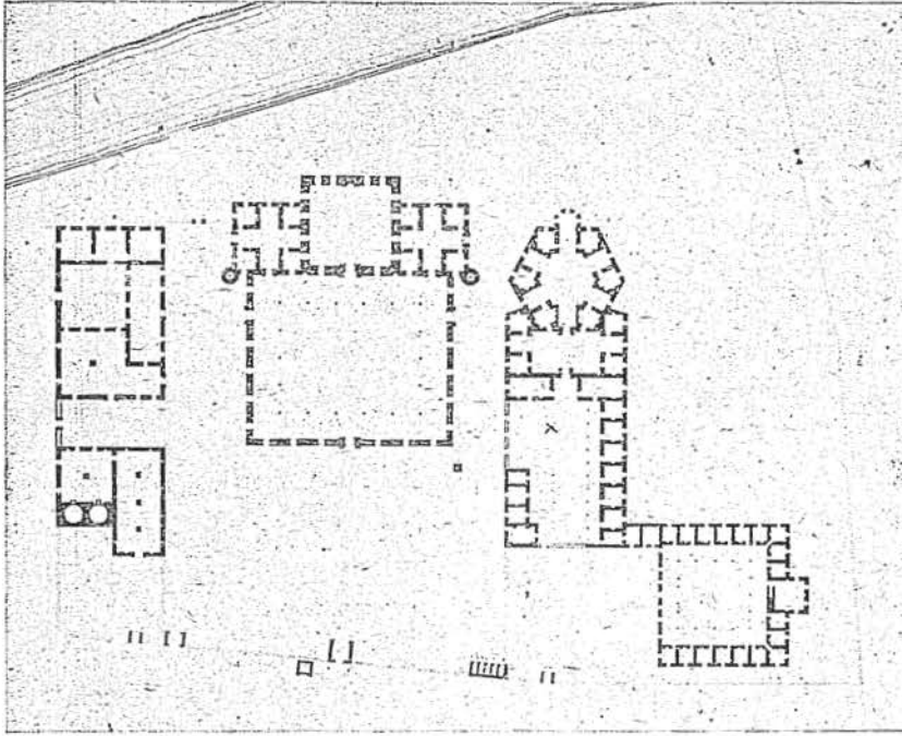
Edirne Darü'ssifasının Bayezit Camii ve Medresesi ve İmareti ile birlikte pılları (Mimar Sedat Çetintaş tarafından çizilmiştir.)
