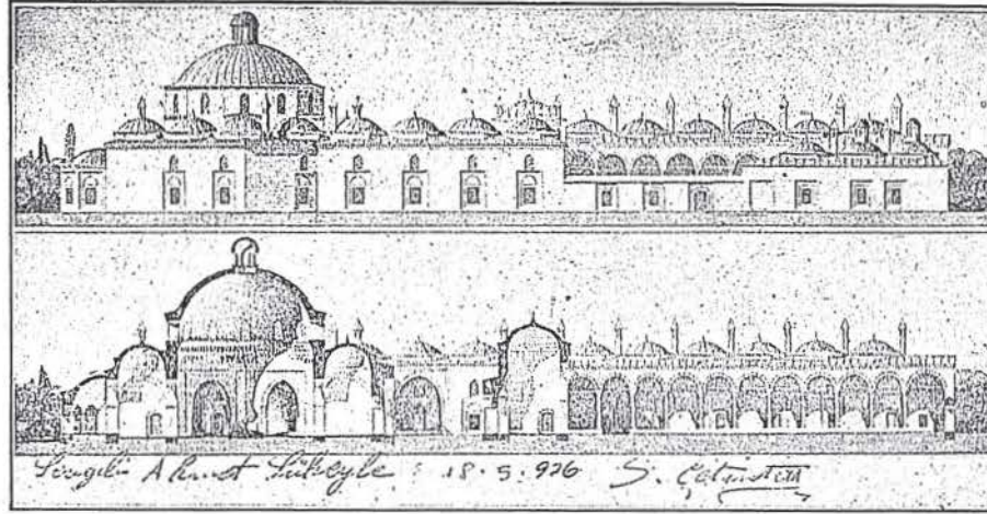
Edirne'de Bayezid II darüşşifasının görünüşü Mimar S. Çetintaş tarafından çizildi.
