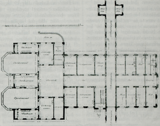
5 — Ameliyat salonlarını ihtiva eden binanın eşas hatları
