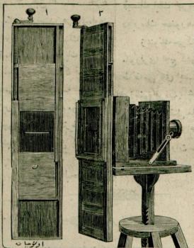
غراب فوطوغرافی - آکانهی فوطوغرافی بو نوع فوطوغرافی اخذ مخصوص اولان آلت
