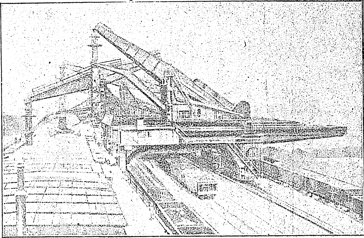
معدن يوكليوب بوشالتيق ايچون قوللانيلان هولت سيستمده اوتوماتيك دهشارزورلردن برى . بوده شارزورلردن الليدن فضله سى حكومات متحده آمه ريقانك بويوك كولار ساحلنده كى ليمانلارنده قوللانيلمقده در
