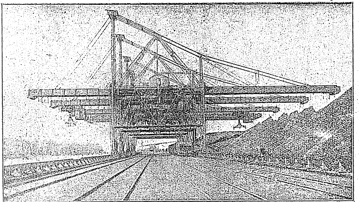
حكومات متحده ده ( اوھيو ) ده ( فھرپور ) ليمانده معدن يوكلك ويا بوشالتيق ايچون قوللانيلان بويوك ويچلر ، بويجه آلتى ماكنه واردر . هر برنك 5 طون يوك آلان برر آغزى بولونور . بو آلتى ماكنه بردن چاليشدينى زمان 10,000 طونلىق بر كمى يوكنى دوت ساعته بوشالتا بيلير . ياز كونلرى بركون ايچنده 10,000 طونلىق ايكي واپورك حوله سنى بوشالتيق ممكندر . بو آلت دنياك الك سريع ايش كورن ده شارزورى صايلير
