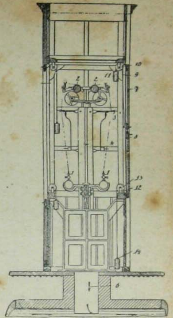
(شکل ۴) ایلیکی بولمک ایچره نوبلرک ماکنسی . (بو، نیتروسلولوز یچین جام ایچنده، مخصوصی برجهازدر . هوا جریانی آشاغیبه دوغوردر . برامه ملومبا واسطه سیله هوا امیلیر .)
