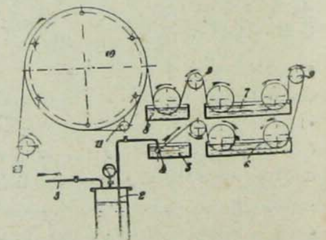
( شکل ۶ ) بسقوز شرکتمک بهراری . بر نومرولوو آشاغیده کی قابده ایپک پلته سی واردر . بوریدن کان هوا تصبیقه بویله ایچ بوریدن جیفیور . صره سیله بیخیلاشمه قانی وسائر محلوللردن کچرک قورومه جرخه واریر .
