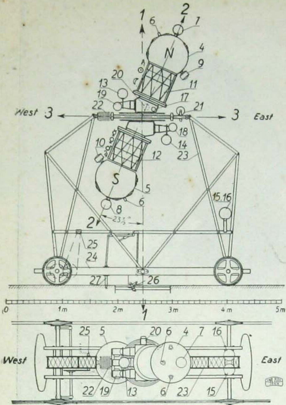
( پلانتهر ) آلنك عرضانى و شاقولى مقطعلرى - آلت بو وضعيتده ايكن شمال قطبنده بولونان بر راصدك سماي نه حالده كوره جكنى عكس اينديرر
