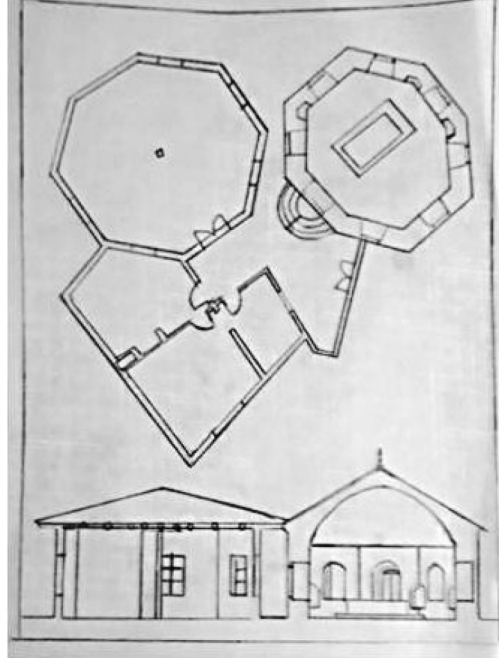
Plan 2: Softa Baba Tekkesi'nin planı ve kesiti (Acar'dan)
