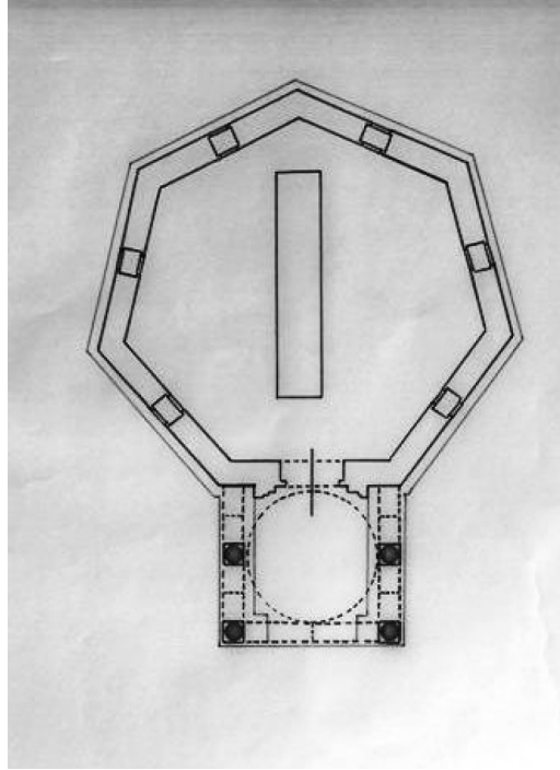
Plan 3: Otman Baba Türbesi'nin planı (Sevgi Parlak'tan)
