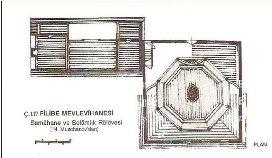
Plan 1: Filibe Mevlevihânesi, semâhâne ve selâmlık
