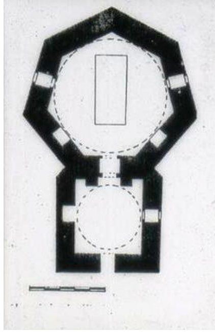
Plan 4: Akyazılı Sultan Türbesi'nin planı (Dürüst'ten)
