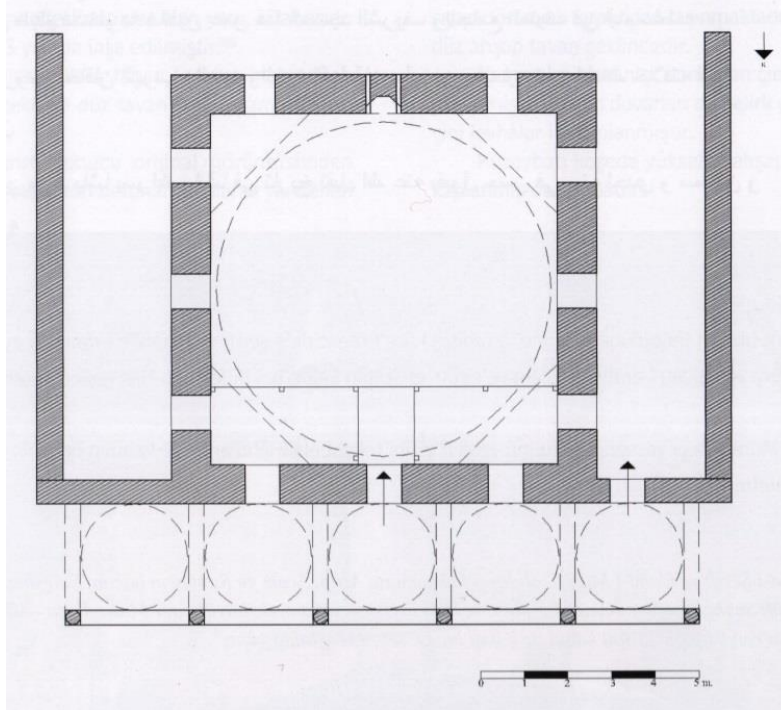
Plan 1 . Erzurum Murat Paşa Cami Planı
