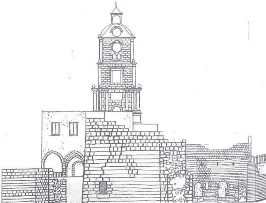
18 Fethi Paşa Saat Kulesi, Kesit (Balducci)
