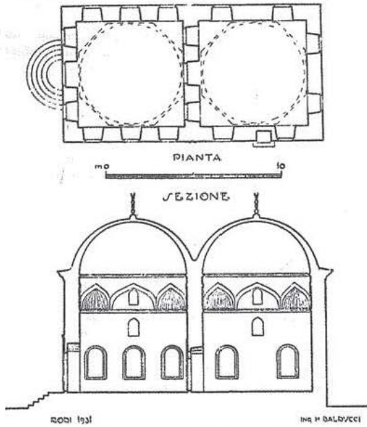
Şekil : 40 — Hafız - Ahmed ağa kütüphanesi (Plân ve makta)
