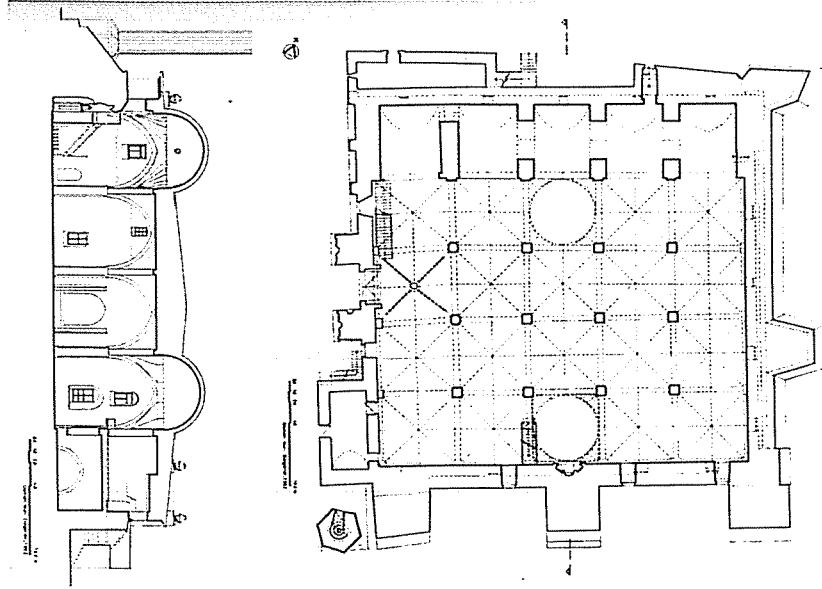
Şekil 1: Aksaray Ulu Camii Plan ve Kesiti (Dülgerler'den)
