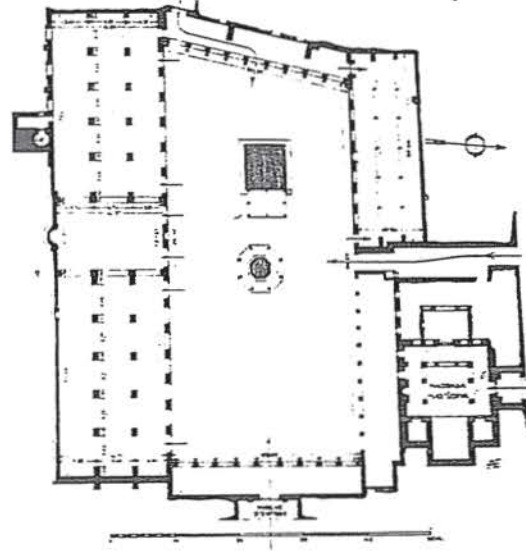
Şekil 14. Düzün planı Gazneliler
