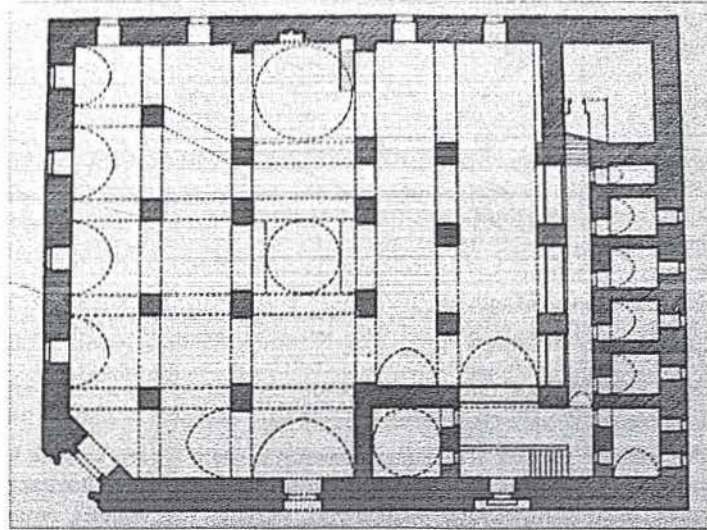
Külük (Gülük) Cami ve Medresesi (Danişmendli-Kayseri-XII.yüzyıl 1135-1142)
