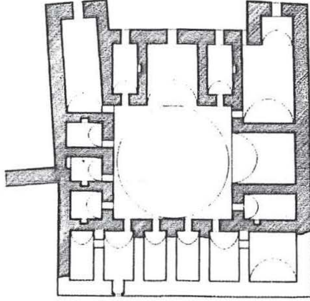
Yağbasan Medresesi Planı Kapalı avlulu ilk medreselerdendir. (Danişmendli-Niksar 1151-1153)
