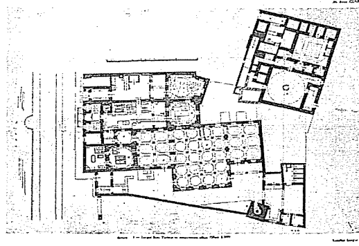
Resim 4. Turgut Reis Türbesi ve diğer yapıların planı (Ölçü: 1/100), Ali Saim Ülgen
