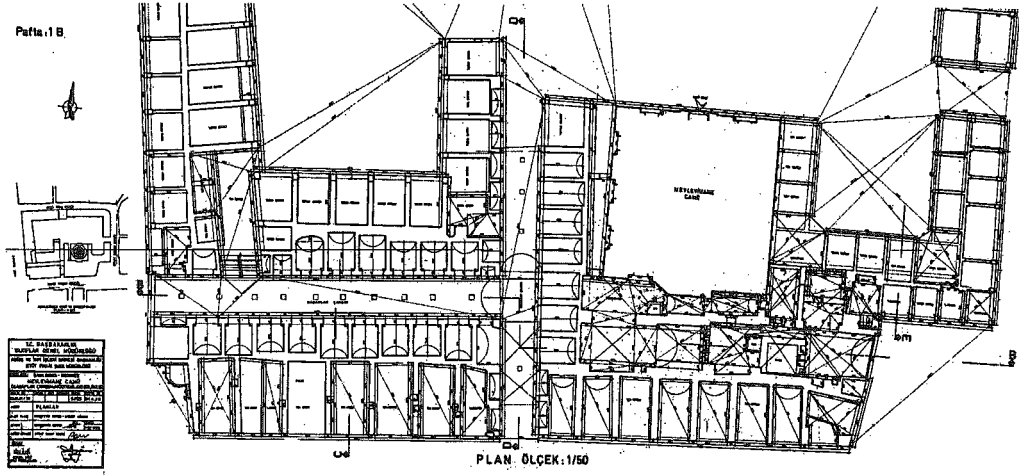
Restorasyon Planlı(Uygulanmayan)
