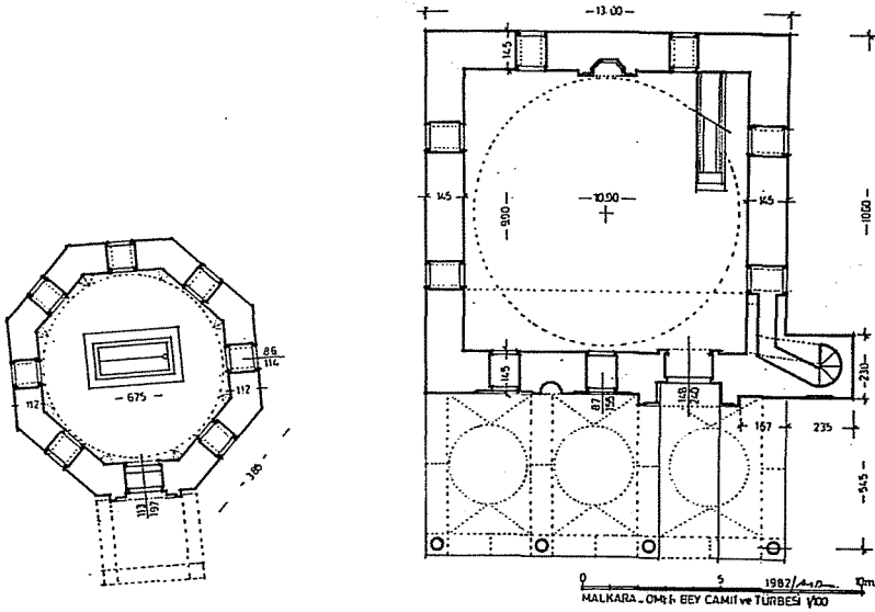
13. Gazi Ömer Bey Camisi ve Türbesi'nin planı (Ayverdi'den)
