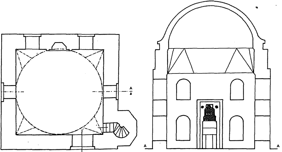
5. Gazi Turhan Bey Camisi'nin planı ve A- A kesiti
