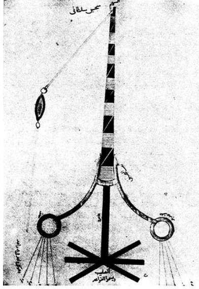
الشكل رقم ١٩ : منجنیق سلطانى ( ص ٤٠ / ب )
