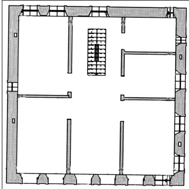
Çiz.4: Selamlık alt kat planı (M.Z. İbrahimgil'den)
