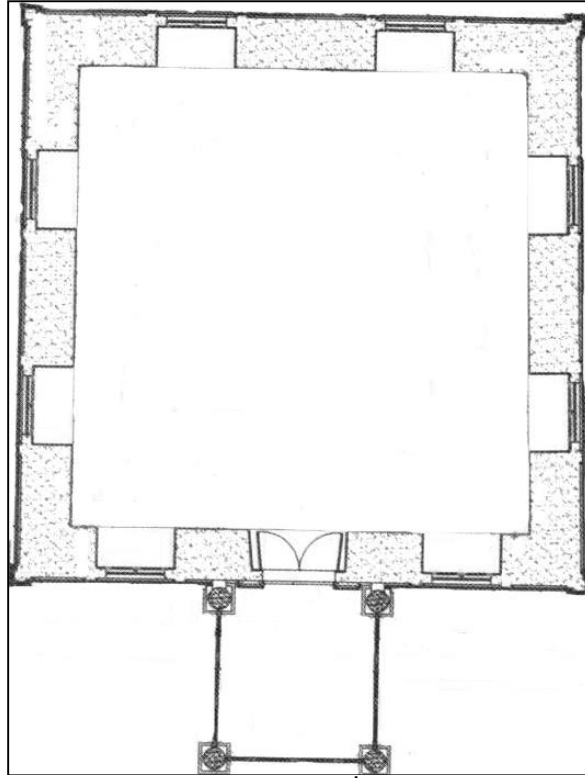
Çiz.2: Türbe planı (M.Z. İbrahimgil'den)
