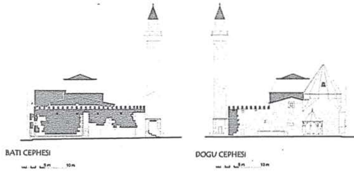
Fot. 14. 1960 onarımı sonrası yapıda görülen değişiklikler (Vakıflar Arşivinde yer alan rölöve çizimleri kullanılarak yapılmıştır)
