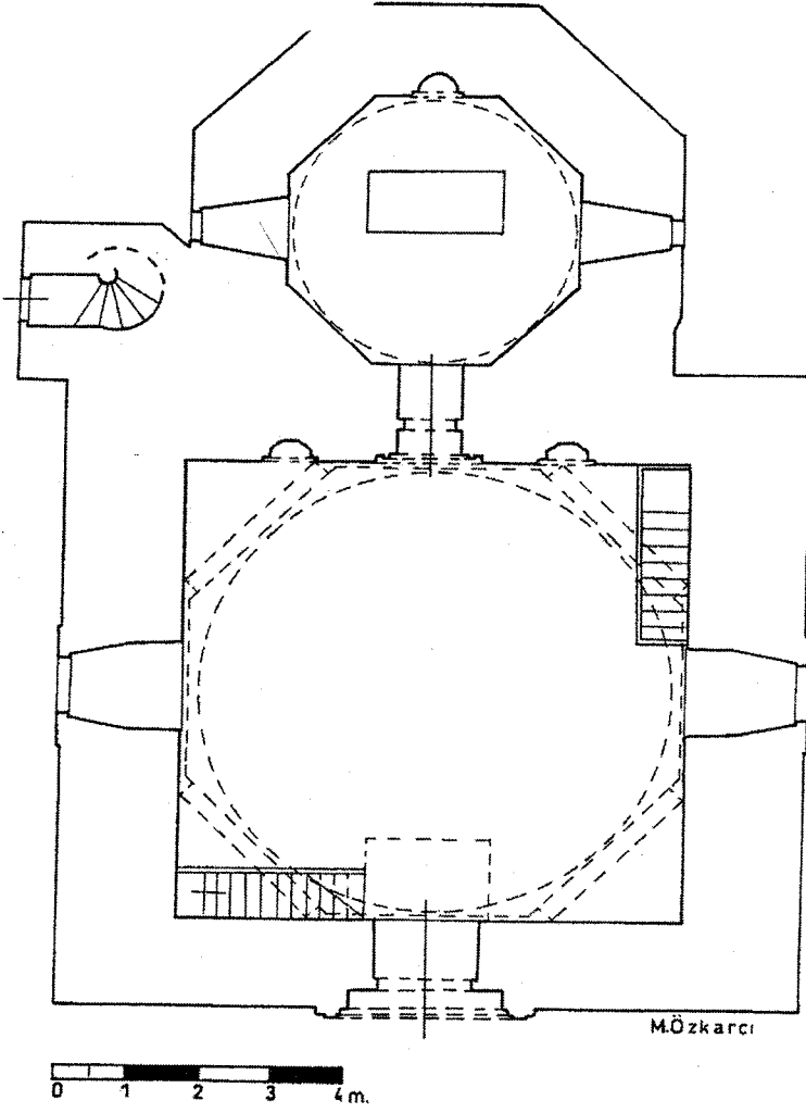
Çizim 1: Elbistan Ümmet (Babaiyye-Hıfnet) Baba Camii ve Türbesi plânı.
