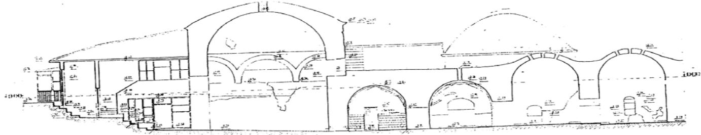
A.A KESİTİ
