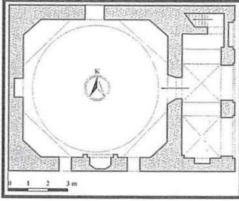
Çizim 1. Haçmaz-Şıhlar Köyü, Şeyh Yusuf Mescidi Plan
