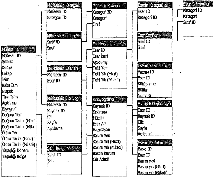
Tefsir Tarihi Veritabanındaki Tablolar ve Birbirleriyle İlişkileri
