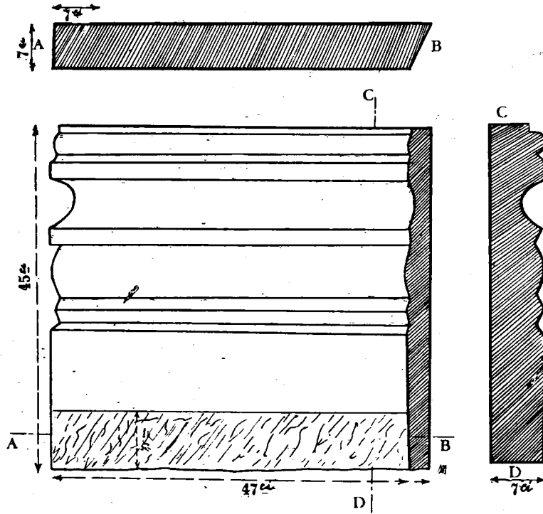
Res. 8 — 1 inci devreye ait mermer duvar sögesi
