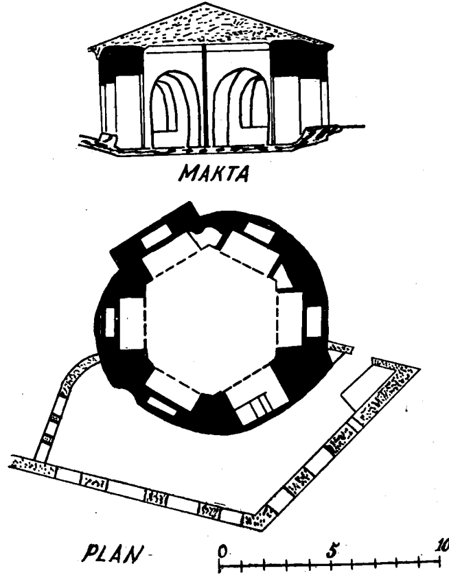
Res. 3 — V. Millingen tarafından yapılmış plân ve makta
