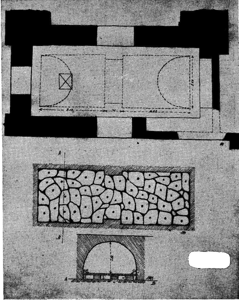
Res. 23 — Yuşa tepedeki kilisenin mezar odası
