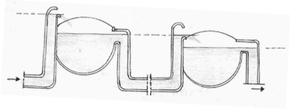
Resim 1: Bileşik kaplar sistemine göre çalışan Bursa çeşmesinin çalışma şeması (Özer, age., s. 30)
