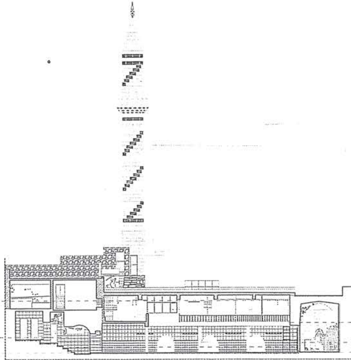
Çizim 5 Şeyh Şeyhullah Camii, B-B Kesiti [Restoratör Mesut Dağgibi-CM Restorasyon Mimarlık, 2017].
