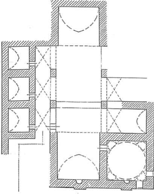
Çizim 20 Sitti Radviyye (Hatuniye) Medresesi, Plan [Altun 1978: 117].
