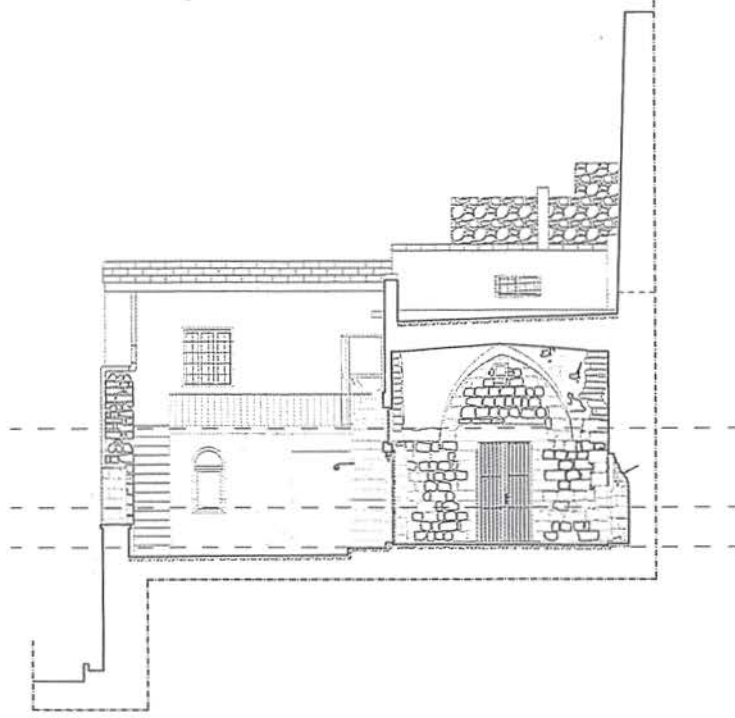
Çizim 13 Şeyh Şeyhullah Camii, J-J Kesiti [Restoratör Mesut Dağgibi-CM Restorasyon Mimarlık, 2017].
