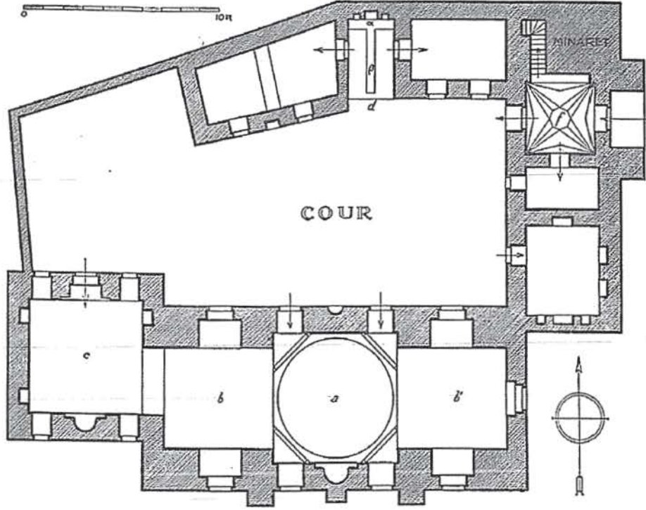
Çizim 18 Melik Mahmud Camii, Plan [Gabriel 1940: 24].
