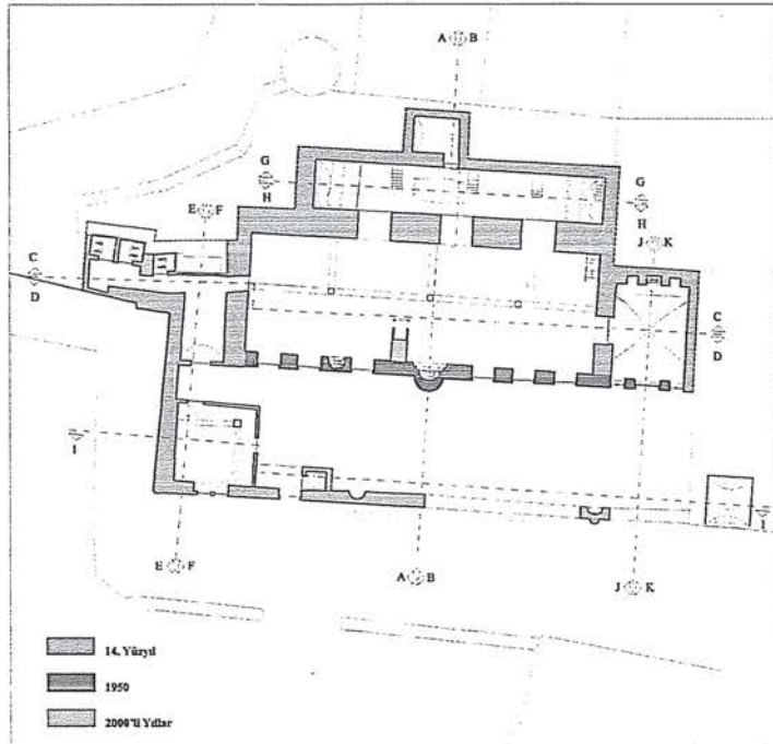
Çizim 2: Şeyh Şeyhullah Camii, Plan, Dönem Evreleri [Restoratör Mesut Dağgibi-CM Restorasyon Mimarlık, 2017.
