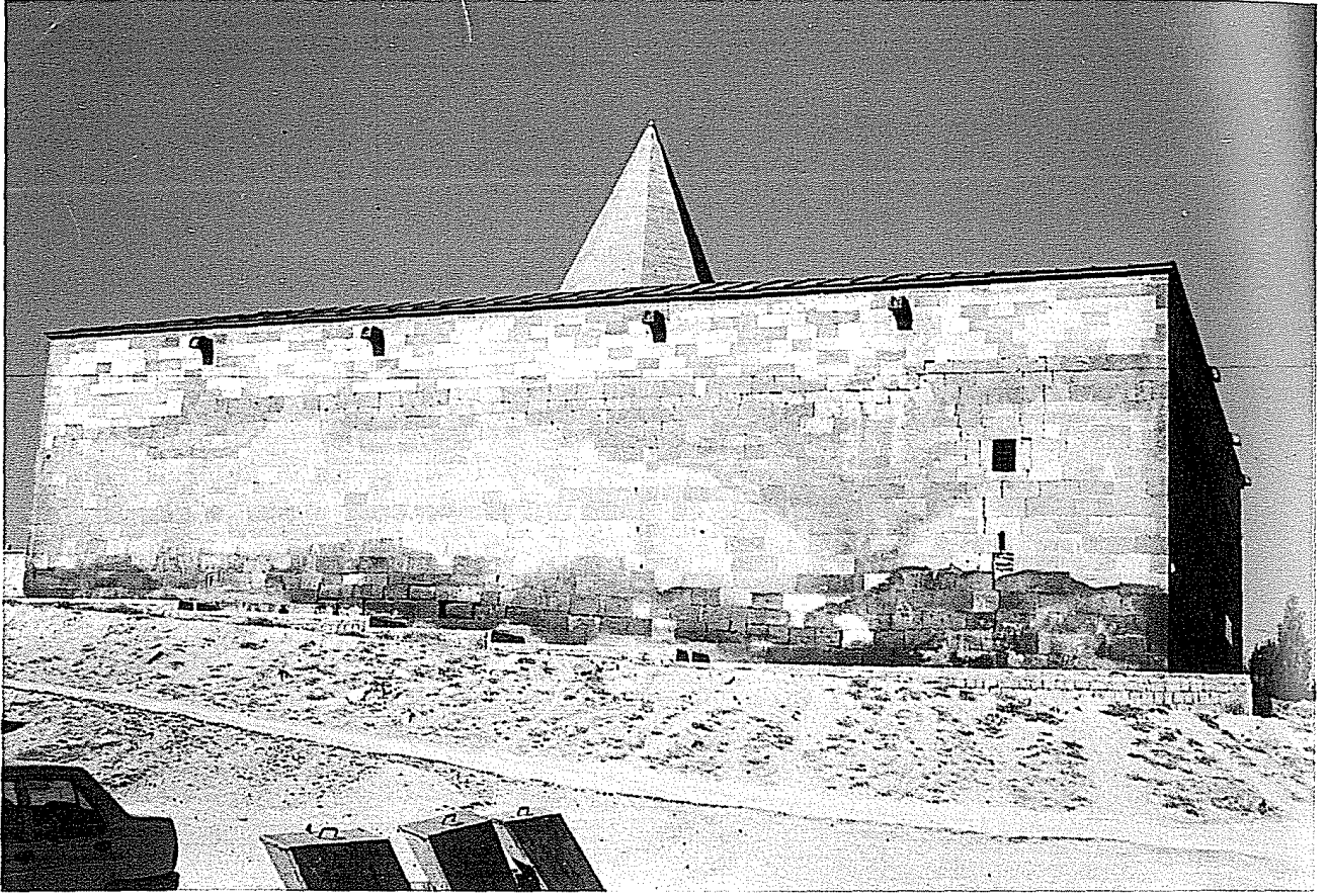
Res. 3: Kayseri Köşk Medrese
