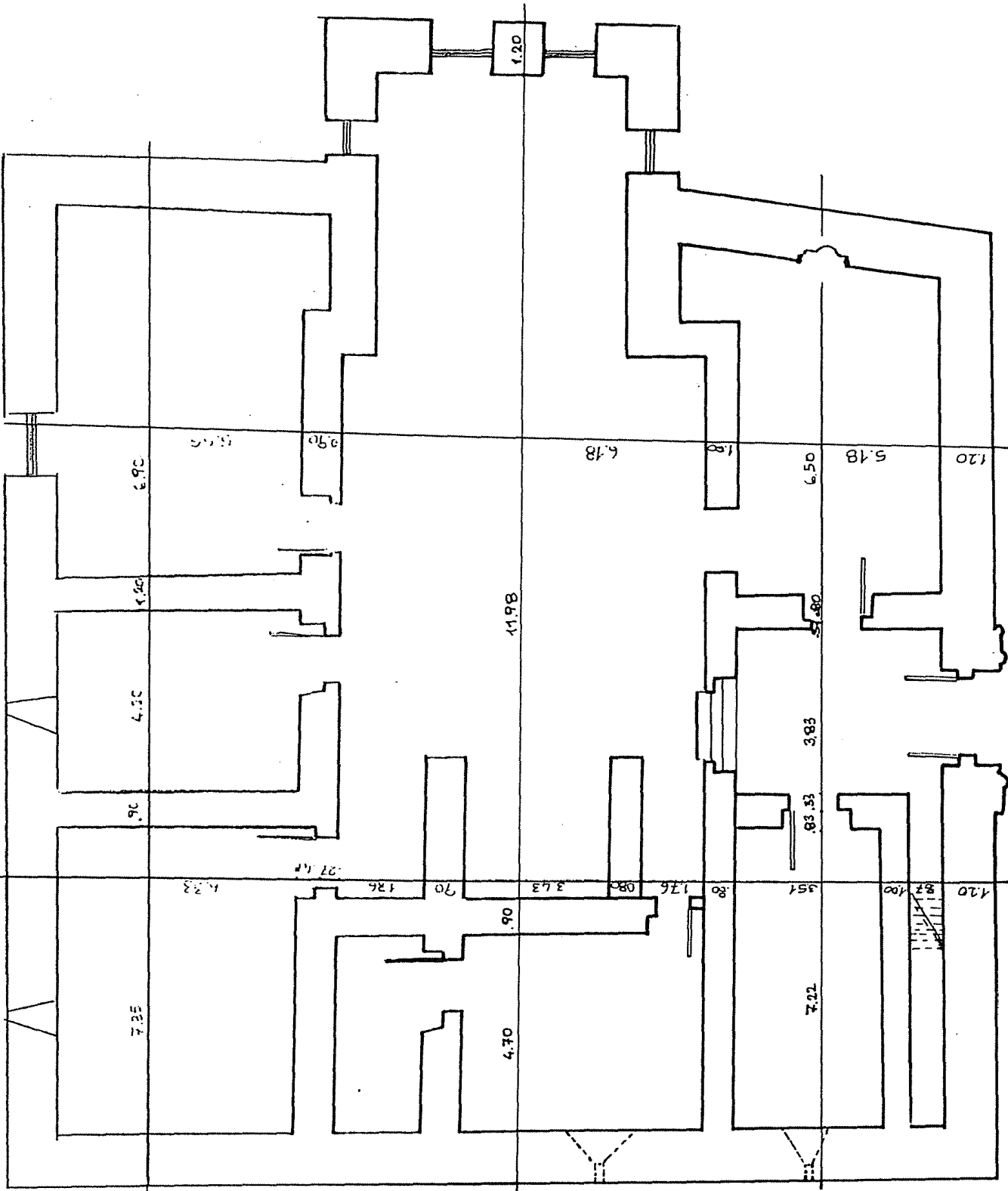
TAŞKINPAŞA MEDRESESI VAZİYET PLANI
