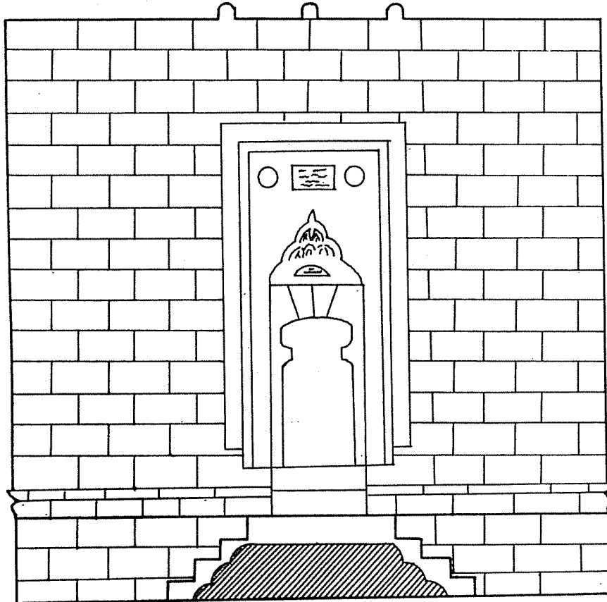
EMİR ŞAHAP TÜRBESİ ÖLÇEK 1/50 ÖN CEPHE GÖRÜNÜŞÜ
