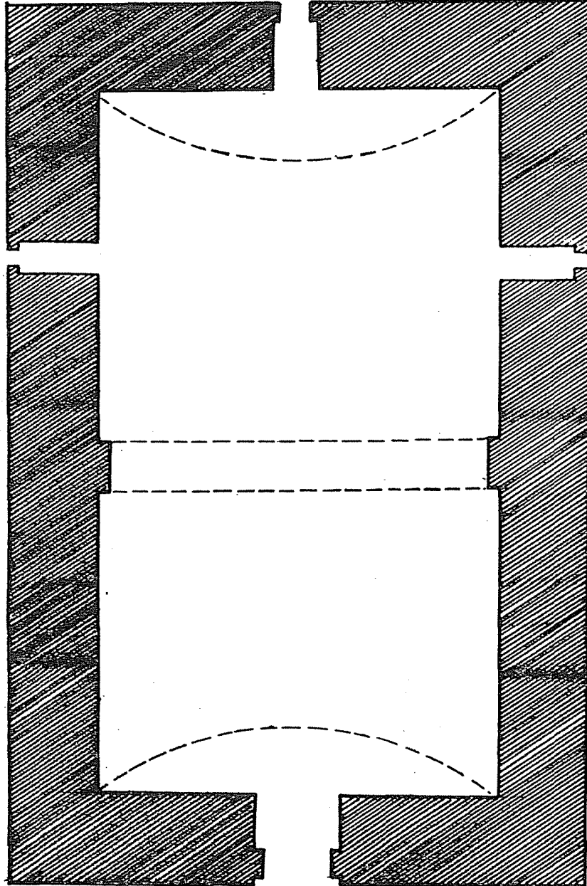
EMİR ŞAHAP TÜRBE PLANI ÖLÇEK 1/75
