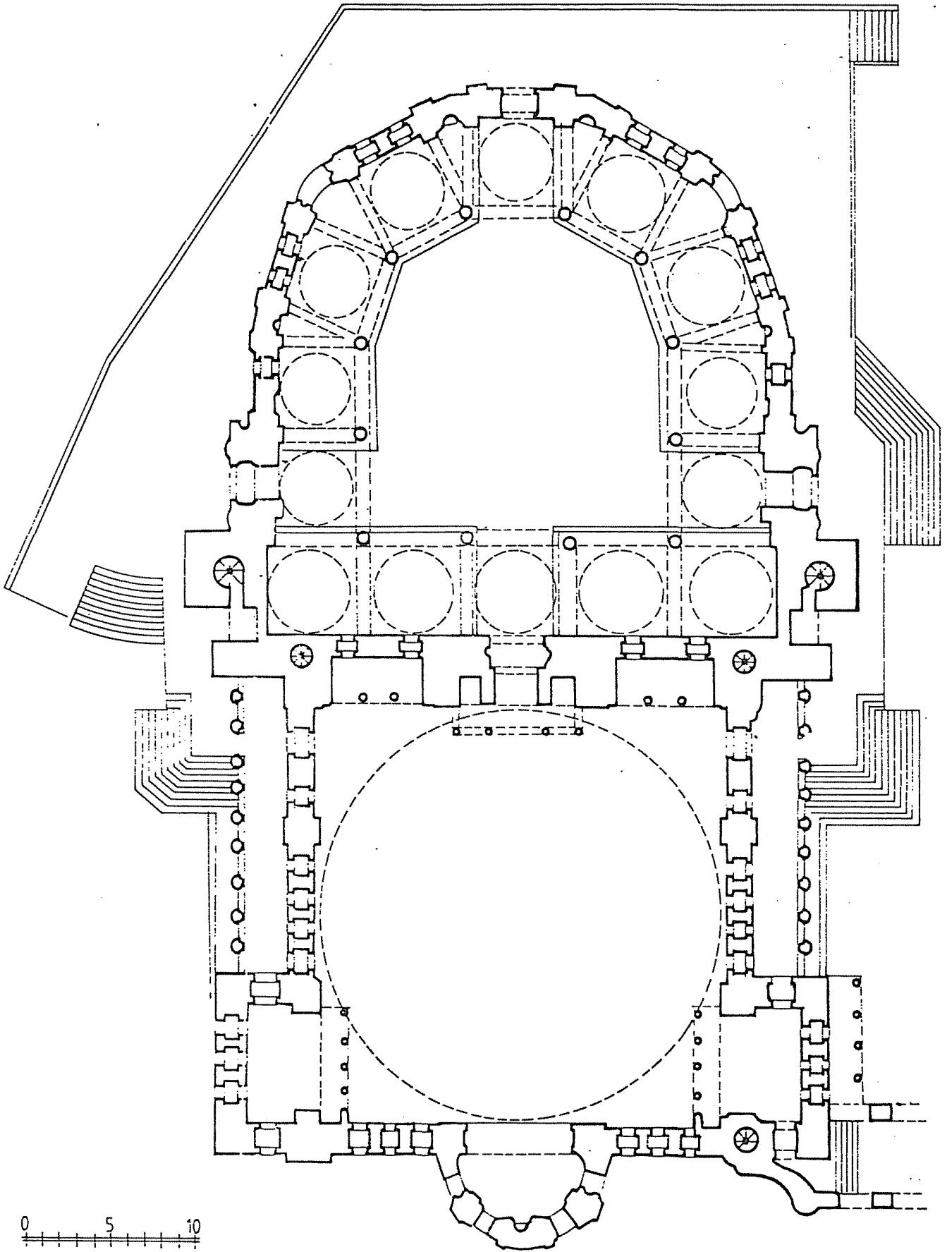
Nuruosmaniye Camii plâni (G. Goodwin'den)
