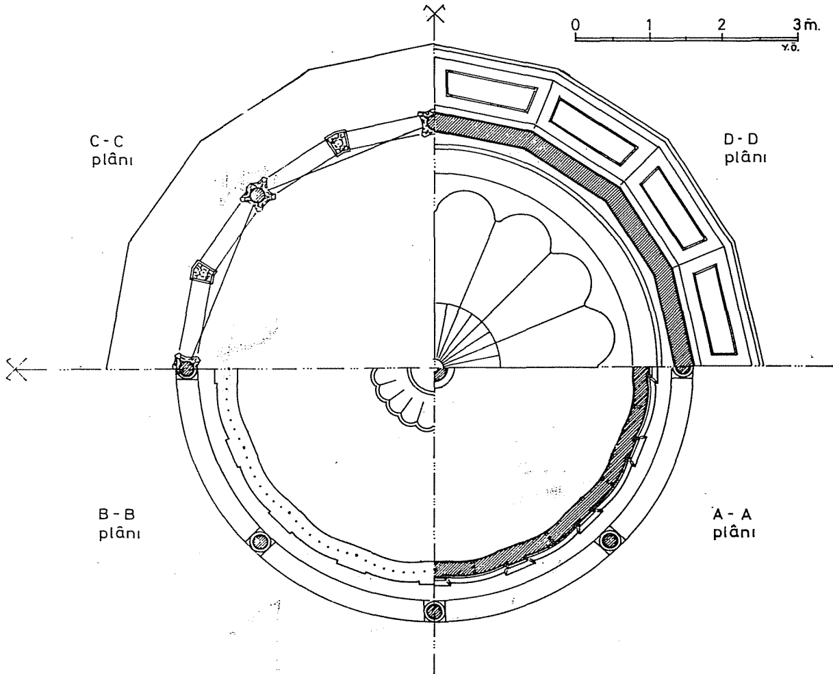
Çizim 1: Mevlana Dergâhı'nın Şadırvanı (Y.Önge'den)
