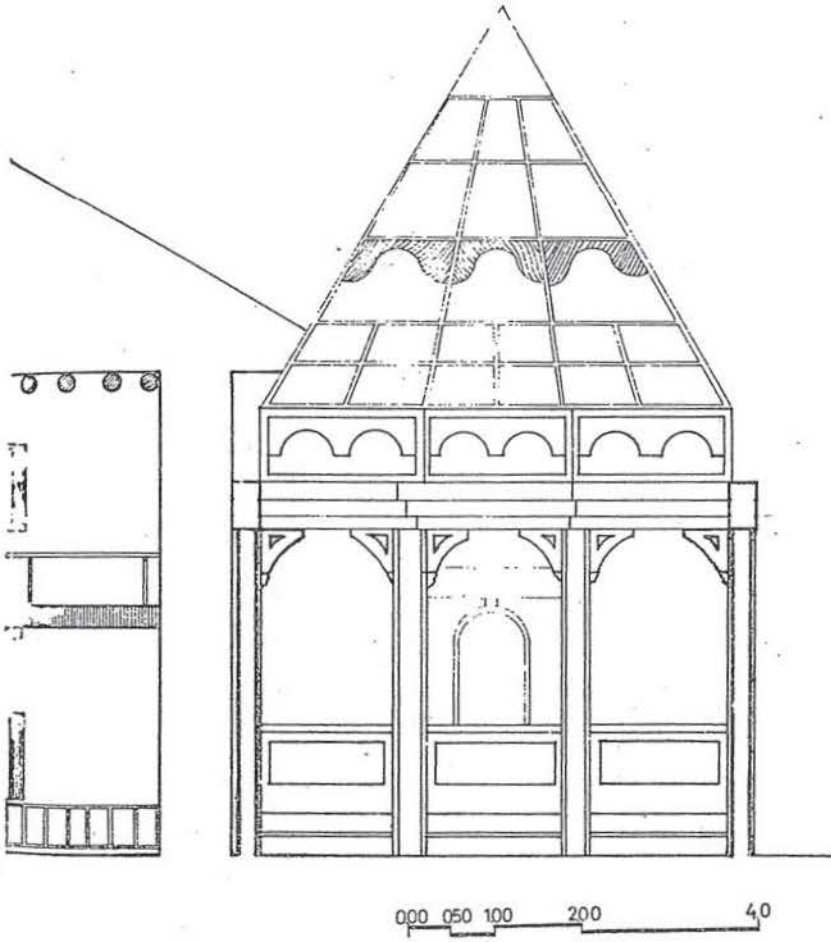
Şekil : 2 — Türbe'nin kesiti (Osman Nuri Dülgerler'den).
