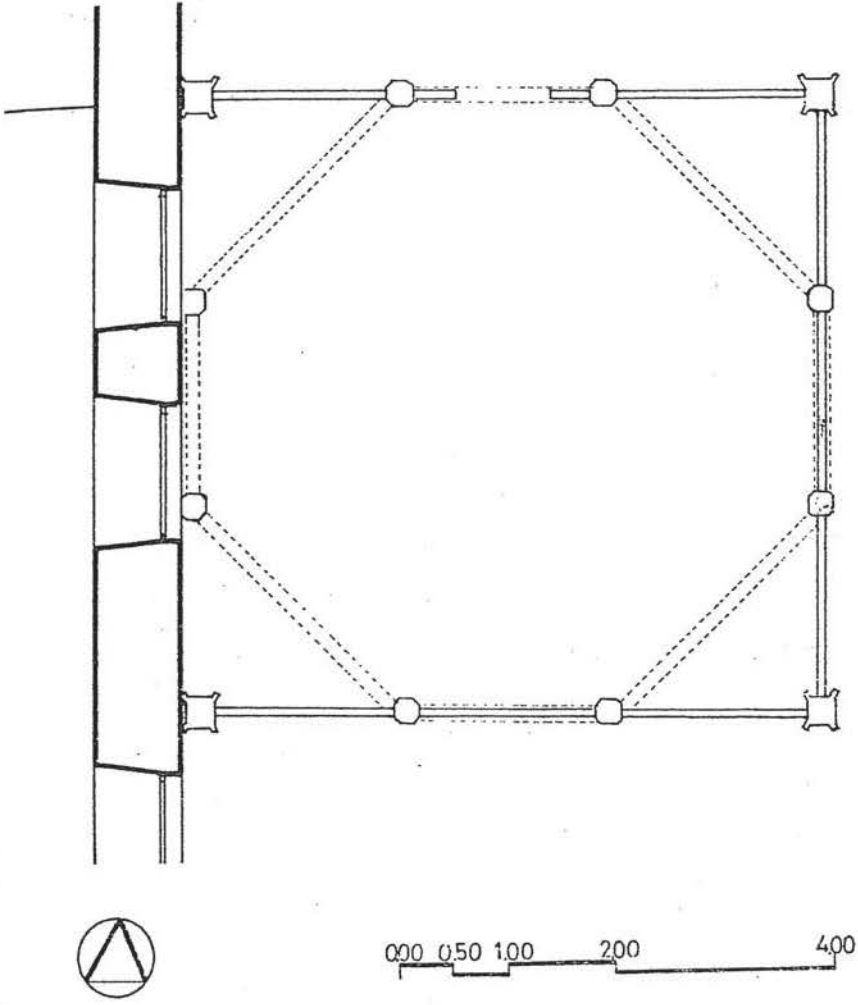
Şekil : 3 — Türbe plâni (O. N. Dülgerler'den).
