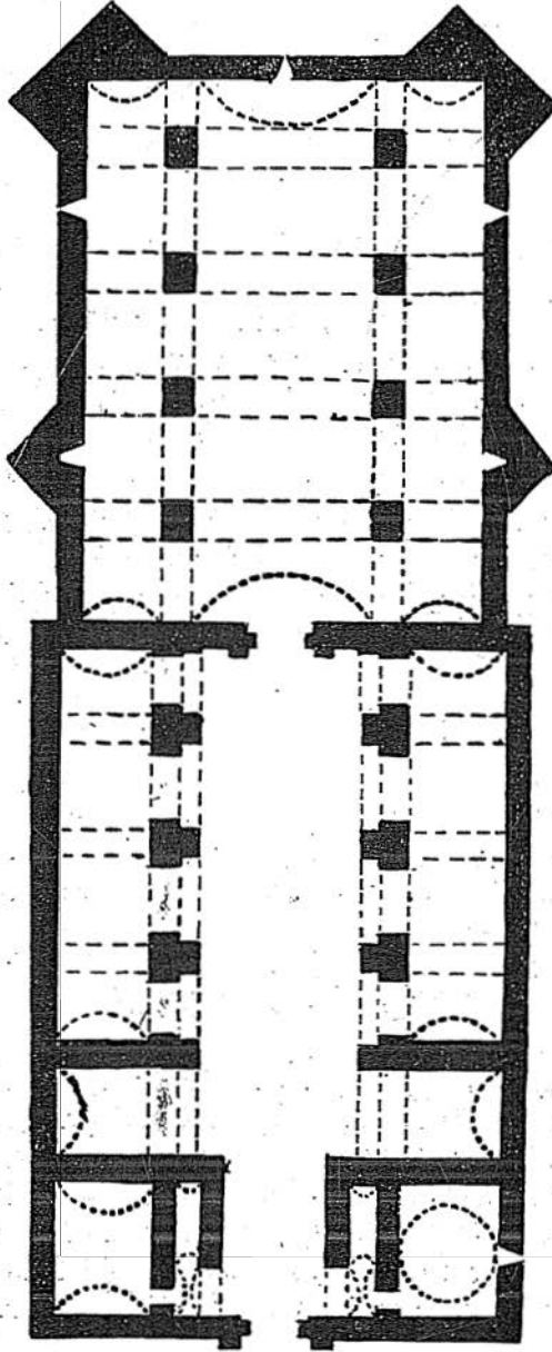
Şekil: 1 — Gelendost: Kudret Hanın plânı.
