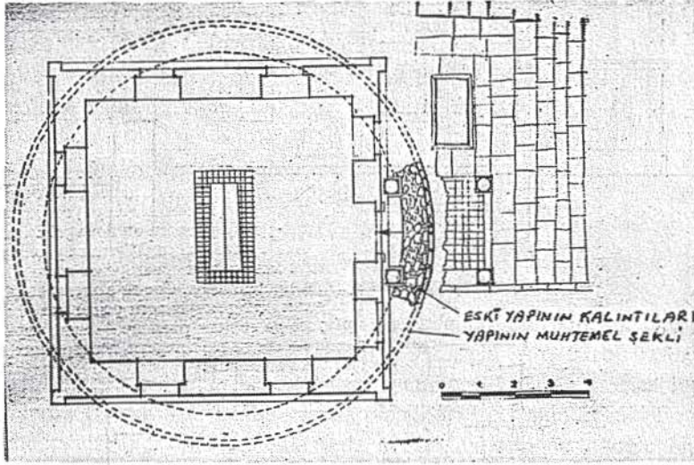
Resim : 5 — Türbenin etrafı ve altında bulunan eski bir yapının temel kalıntıları plânı (M. Lukic)
