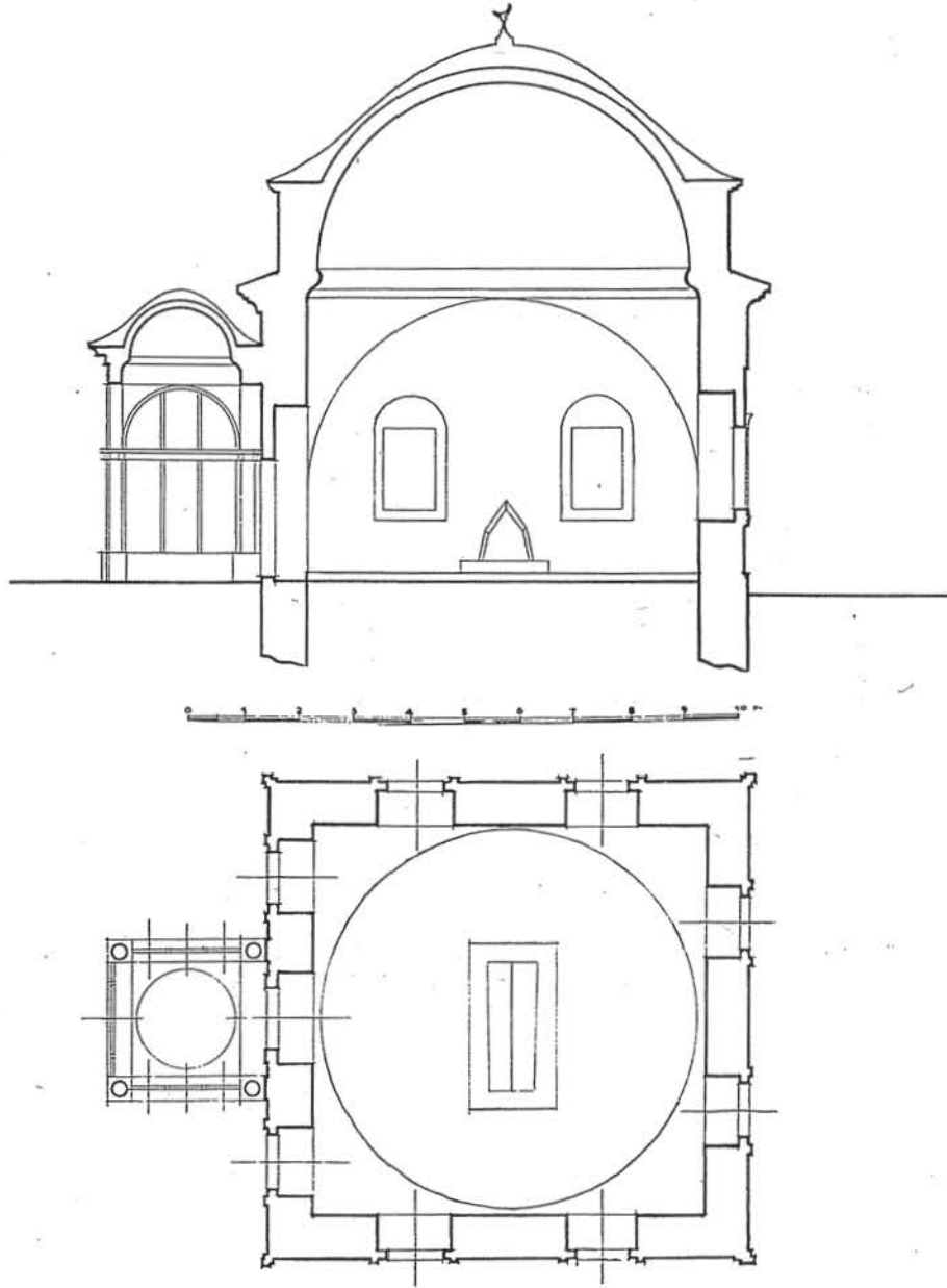
Resim : 6 — Kosova'da I. Murat türbesinin plân ve kesiti (I. Zdravkoviç)
