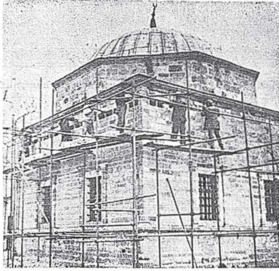
Resim : 4 — Kosova'da I. Murat türbesinin 1960-1961 yıllarındaki onarımı (M. Lukiq'ten)
