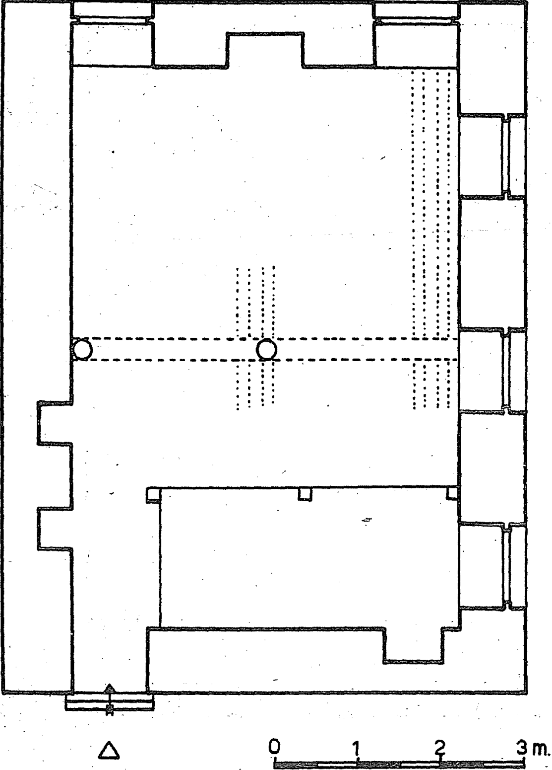
4. Şekil: Kamerolu (Taşbaşı) Mescidi Plânı
