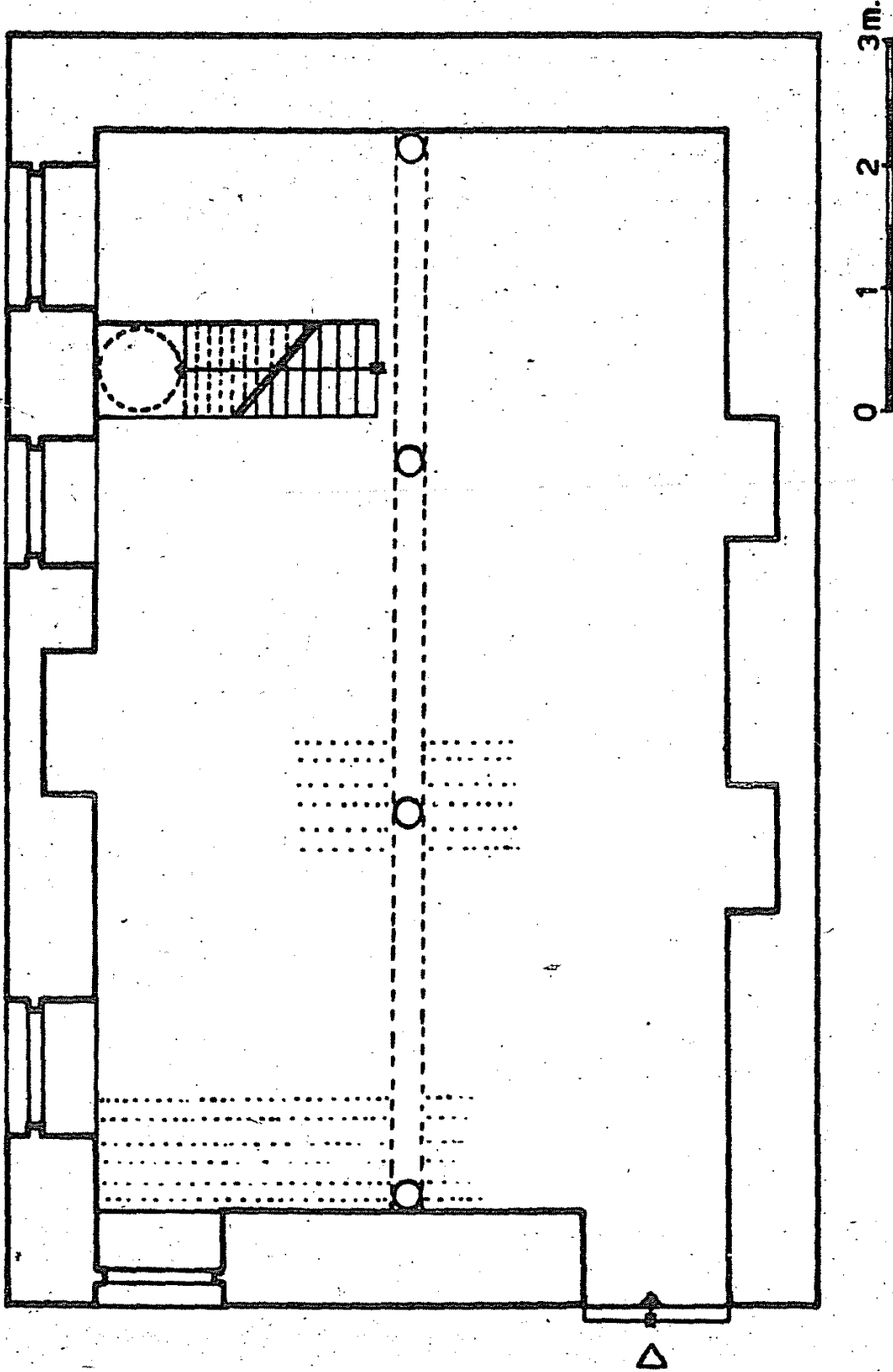
6.Şekil: Aşağı Mahalle Mescidi Planı
